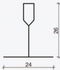
CROSS TEE ( T-24)
